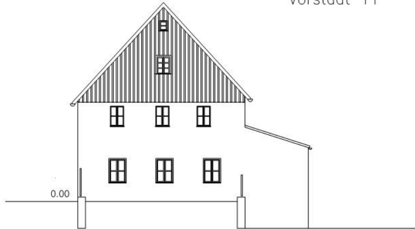
Ansicht Osten
