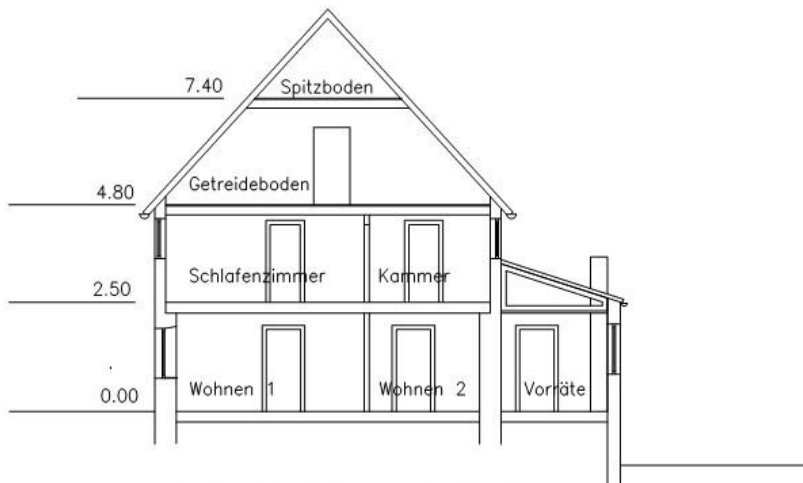
Schnitt Wohnen/Schlafen
